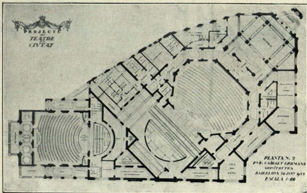
PROYECTO DE «TEATRE DE LA CIUTAT». — PLANTA.
