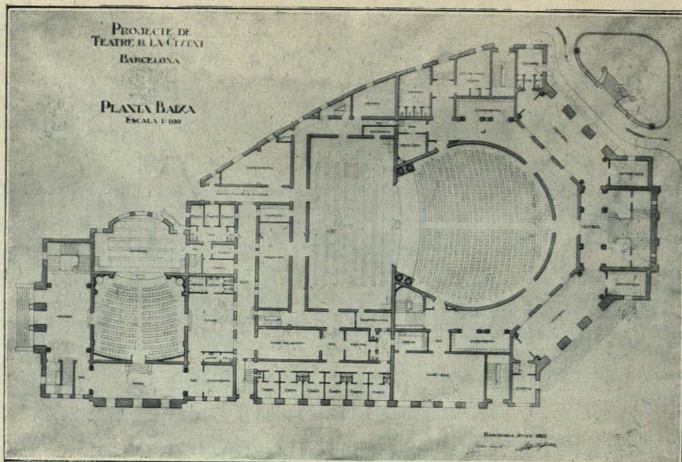
PROYECTO DE «TEATRE DE LA CIUTAT». — PLANTA BAJA.
