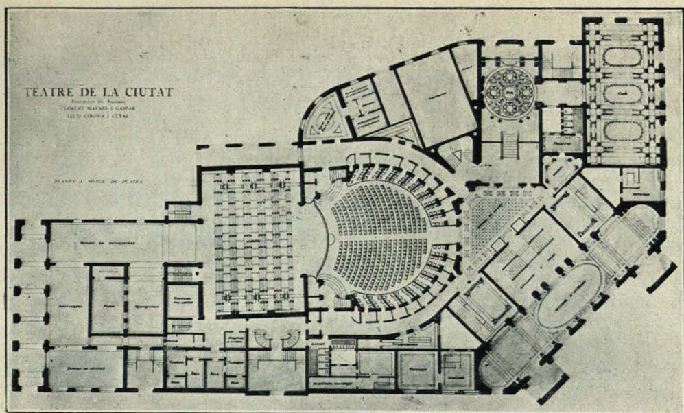
ANTEPROYECTO DE «TEATRE DE LA CIUTAT». — PLANTA DE PLATEAS.
