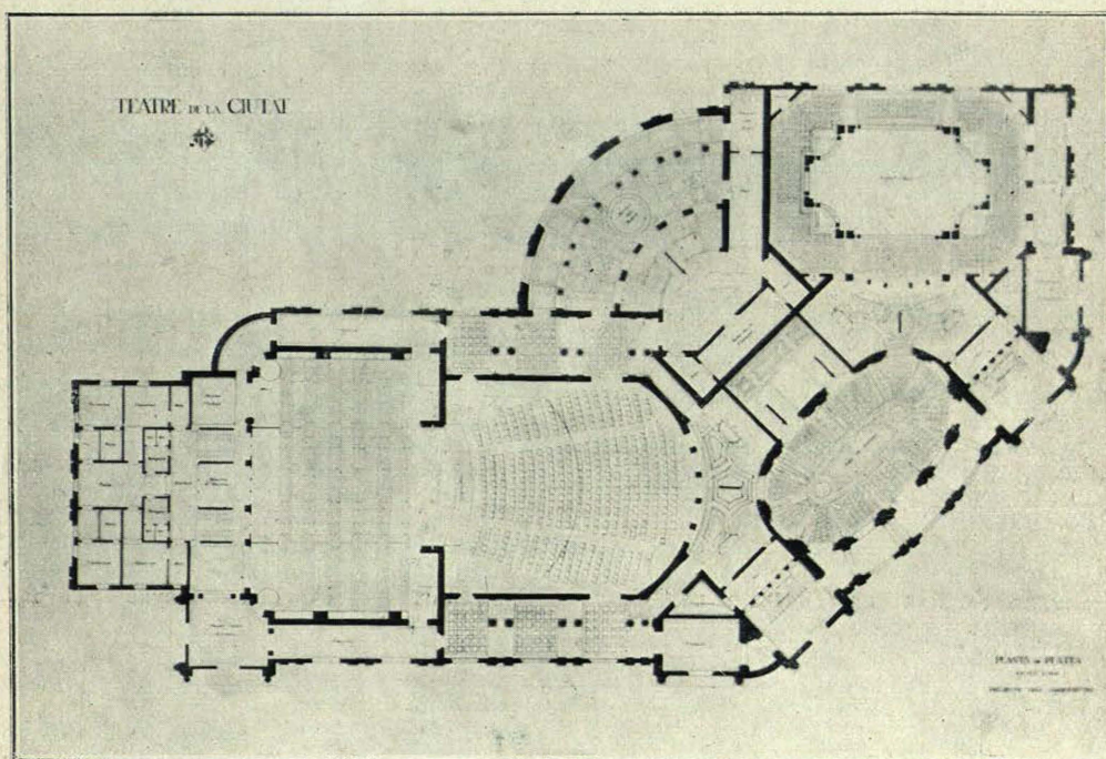
PROYECTO PREMIADO DE «TEATRE DE LA CIUTAT». — PLANTA DE PLATEAS.
