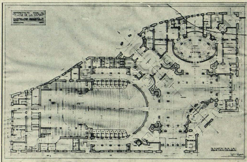
ANTEPROYECTO DE «TEATRE DE LA CIUTAT». — PLANTA BAJA.
