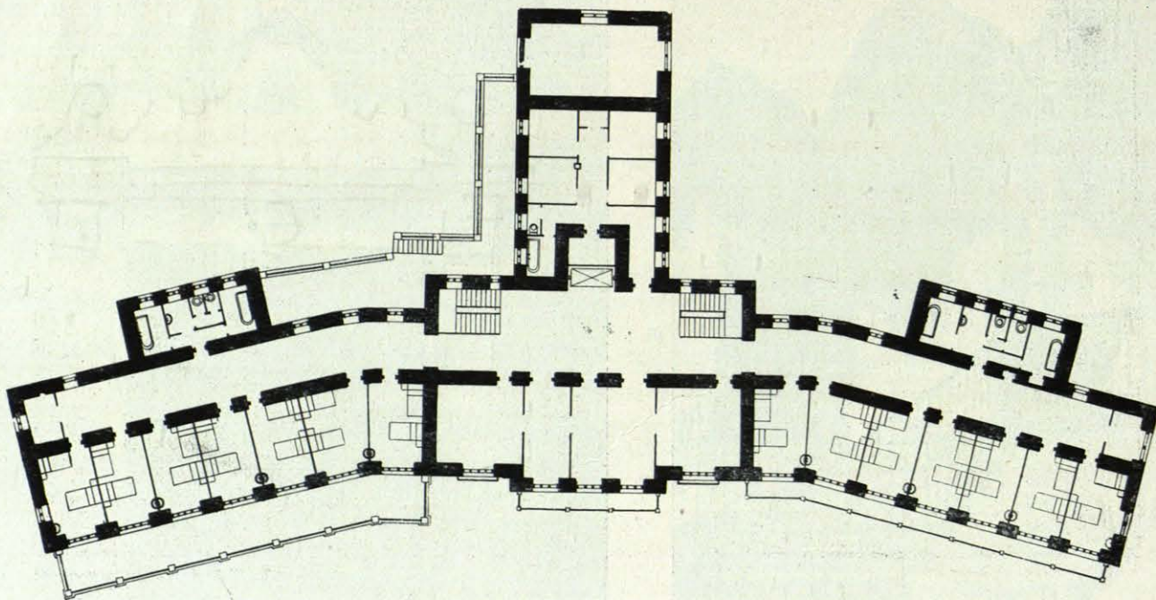
PLANTA DEL EDIFICIO DEL FONDO (OBRA DE 1924).
