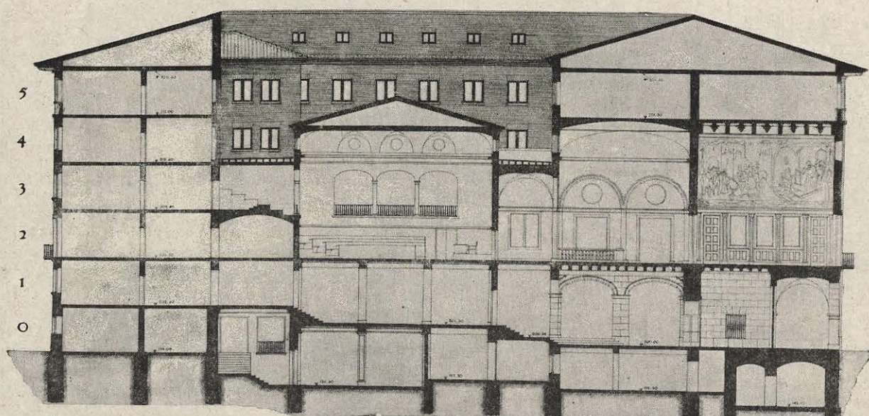
SECCION C-D ESCALA 1:100
