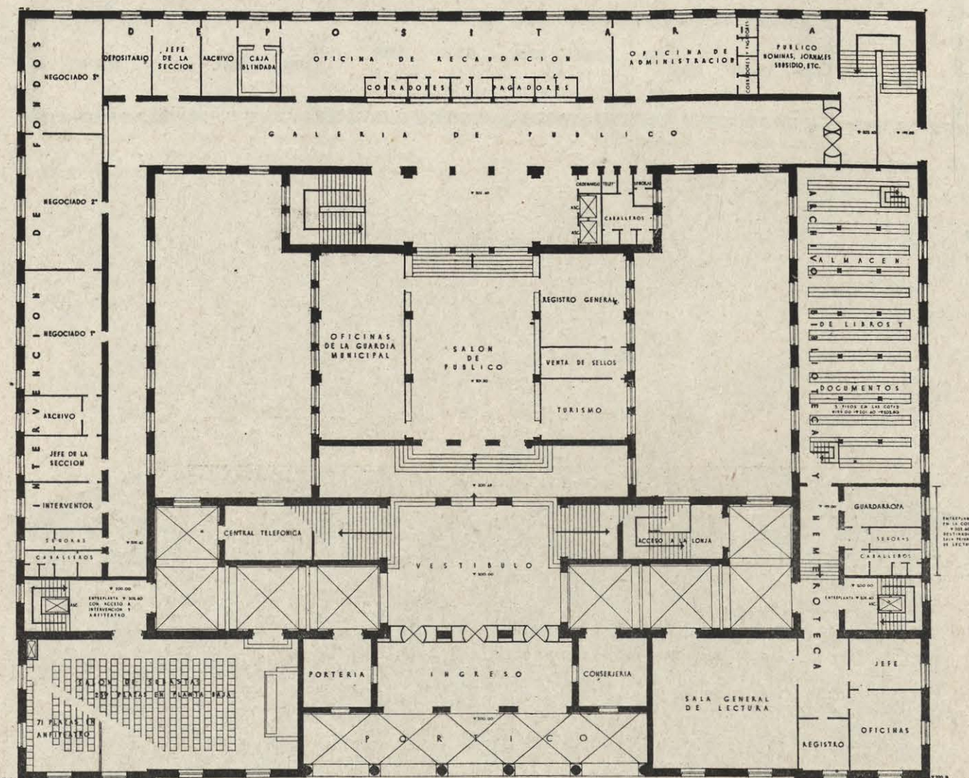
PLANTA 1
