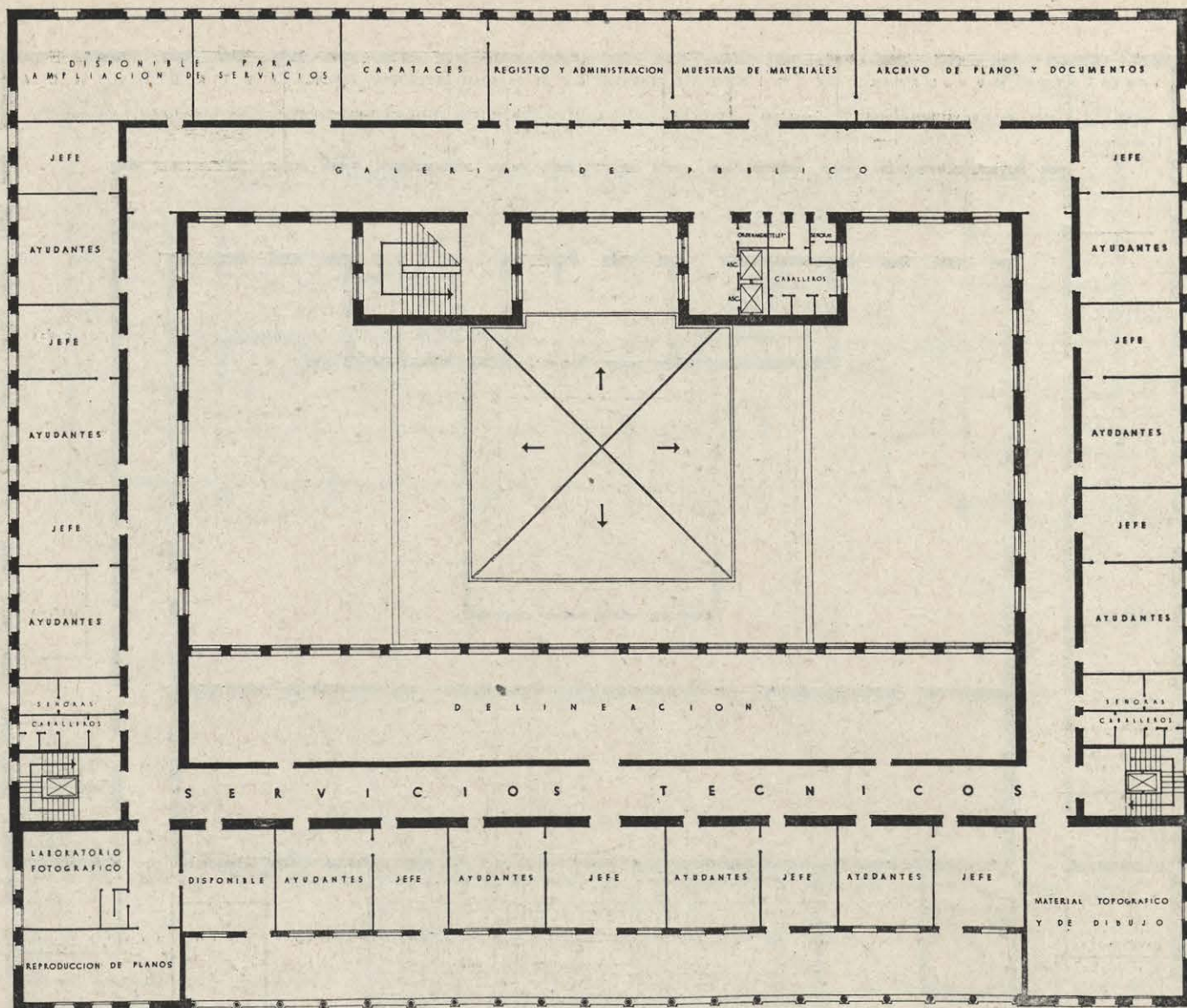
PLANTA 5
