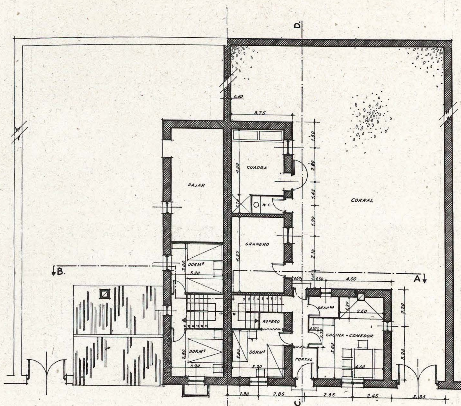
PLANTA ALTA
