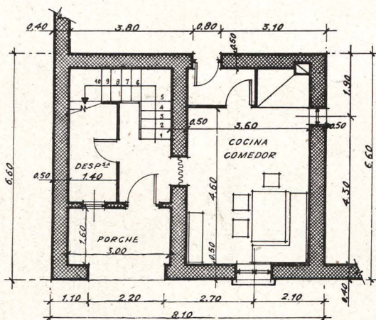
P. BAJA
