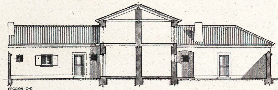
SECCIÓN C-D
