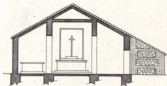
SECCION A:B
