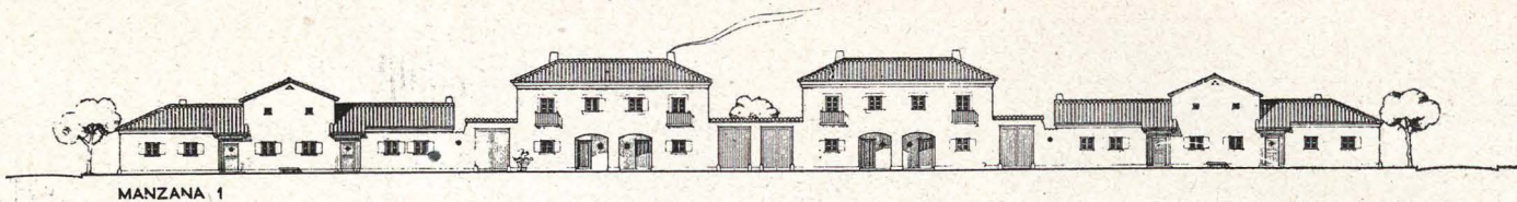
Alzado general de la manzana núm. 1.
