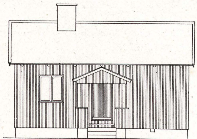
Viviendas para familias de ex combatientes en Finlandia. Tipo A-1. La planta del ángulo inferior izquierdo es la del tipo inferior A-4.
