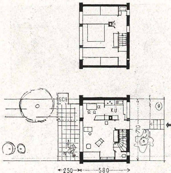
Plantas principal y baja.
