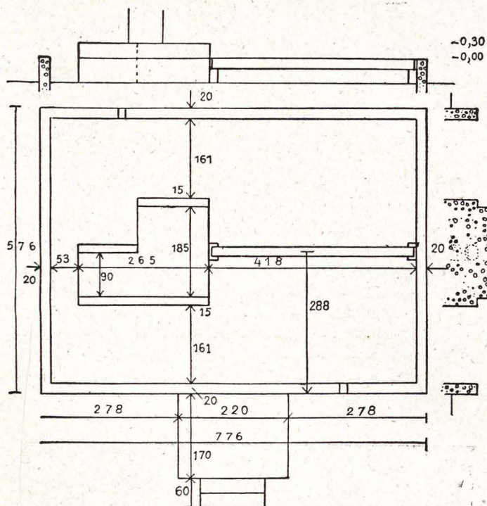
Viviendas para familias de ex combatientes en Finlandia. Tipo A-1. La planta del ángulo inferior izquierdo es la del tipo inferior A-4.
