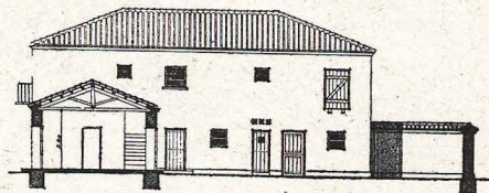
SECCIÓN C-D
