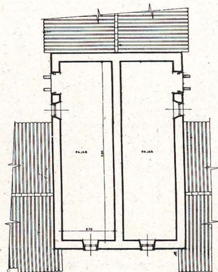
PLANTA ALTA
