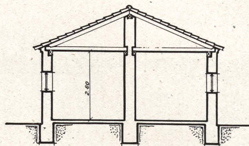
SECCION C-D
