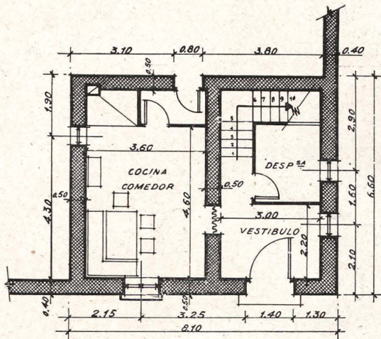
P. BAJA
