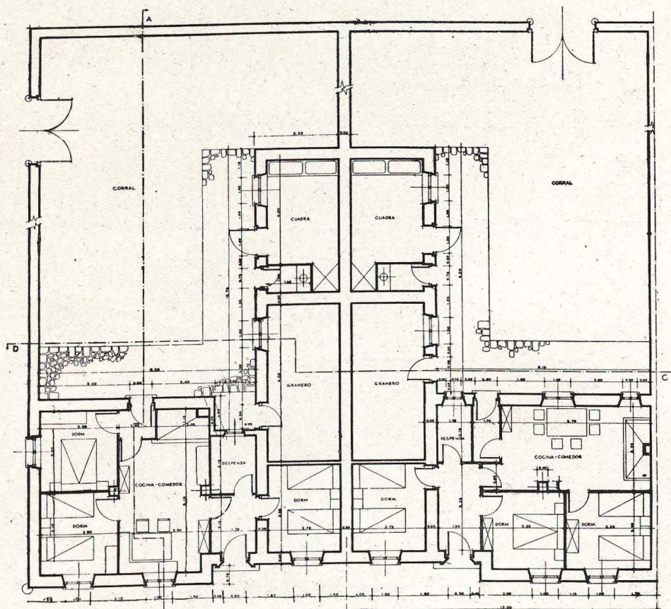
PLANTA BAJA
