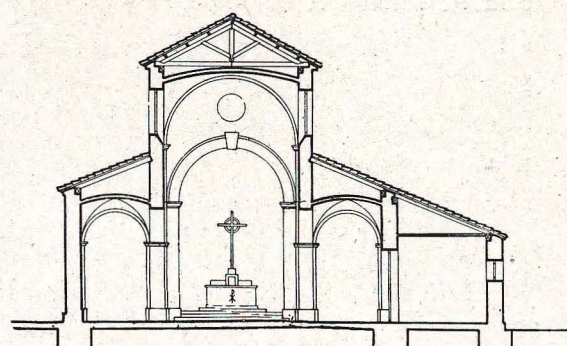
Sección.
