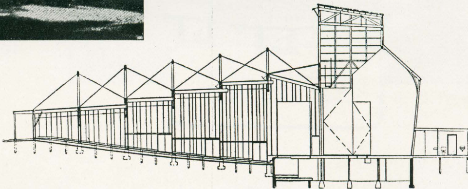
Sección longitudinal y planta.
