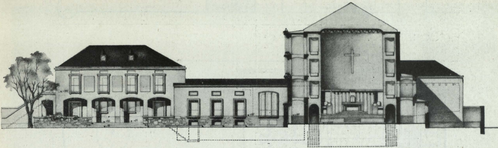
Sección por la nave de la iglesia.
