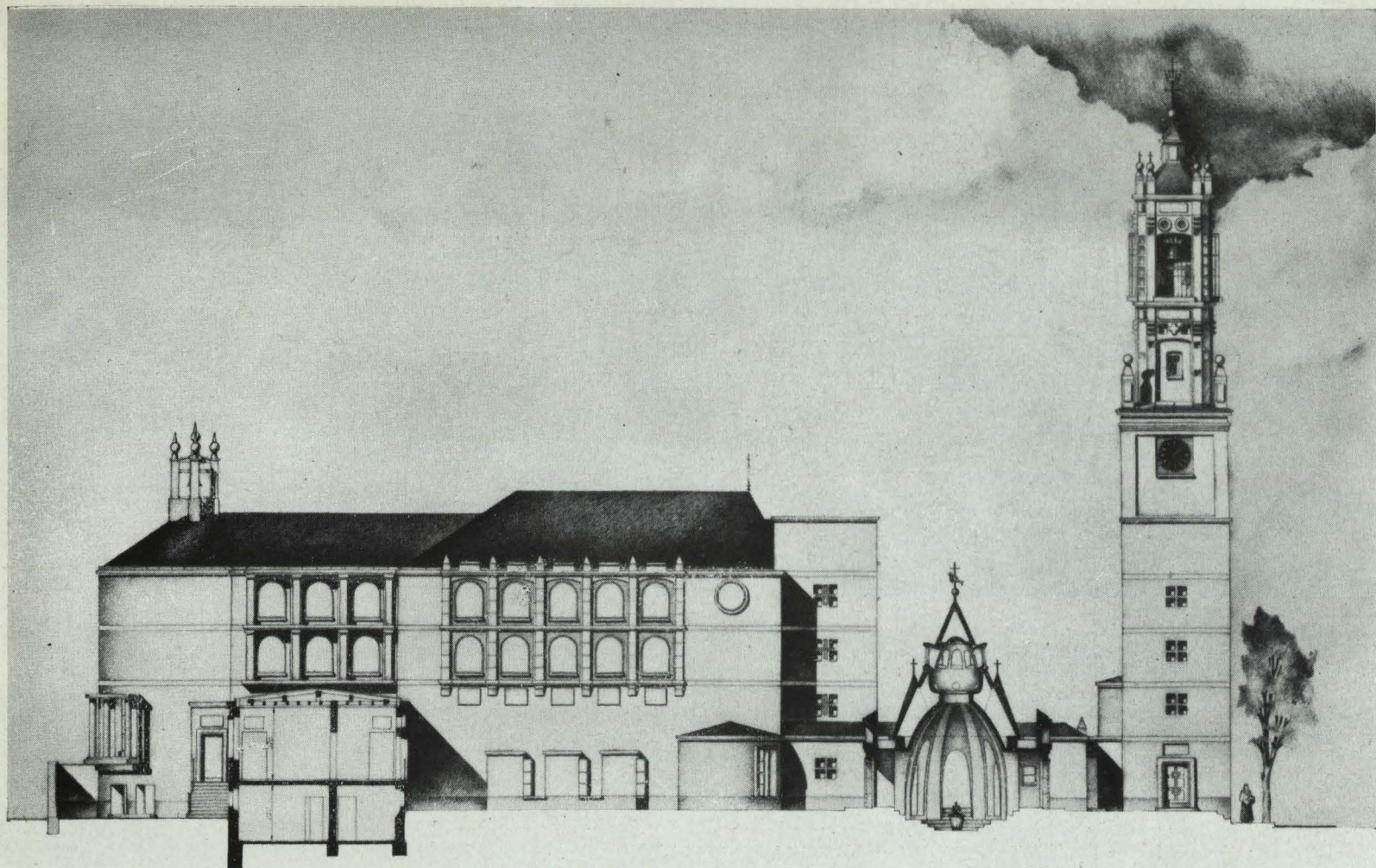
Sección por el Baptisterio.
