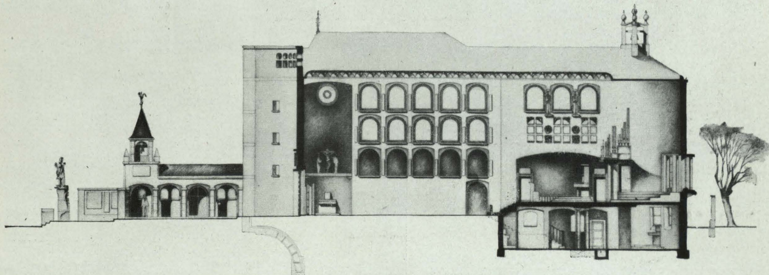
Sección por la nave de la iglesia.
