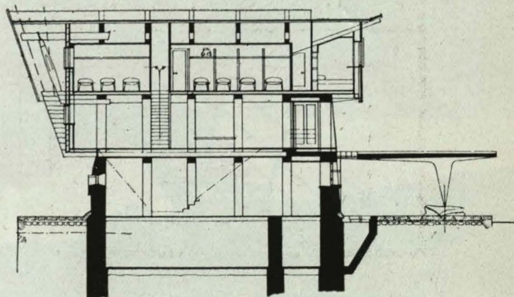
Sección transversal.
