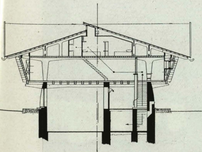
Sección longitudinal.
