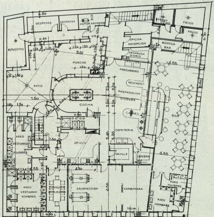
Planta de semisótano.
