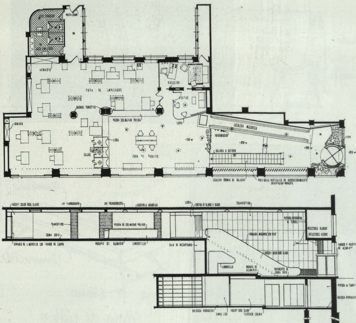
Planta y sección de una Sucursal del Banco Español de Crédito en Madrid. Abajo, detalle de la escalera y pormenor de los mostradores.
