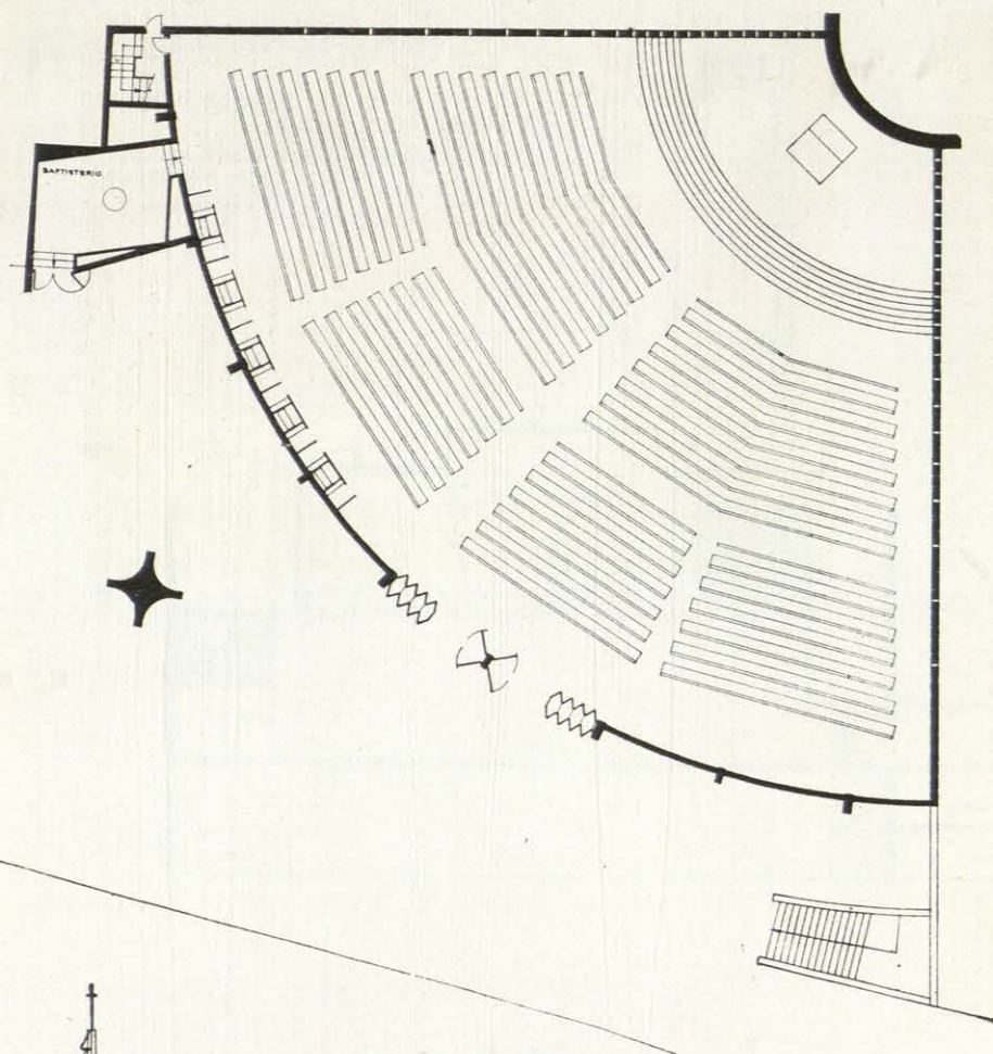
Plantas, sección y detalles del proyecto del arquitecto Miguel Fisac.
