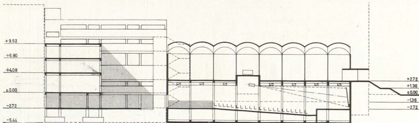
SECCION LONGITUDINAL
