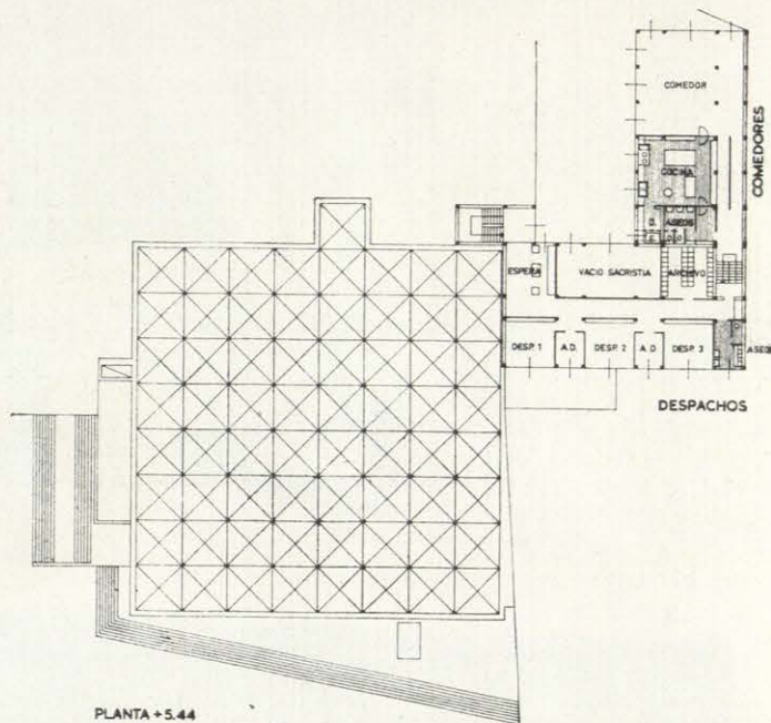
PLANTA +5.44
