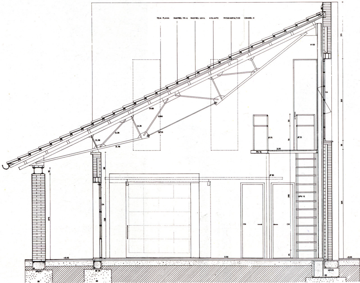
Sección constructiva del taller.
